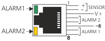
Câblage interne des OPTO MOS
